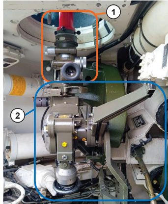
Рисунок 1.6 – Механічний приціл
